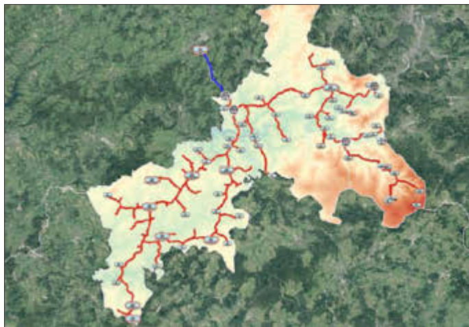
Die „Schlagadern“ der Wasserversorgung im Kreis Altenkirchen. Das Fernleitungsnetz des WKA umfasst 230 Kilometer. Foto: WKA
